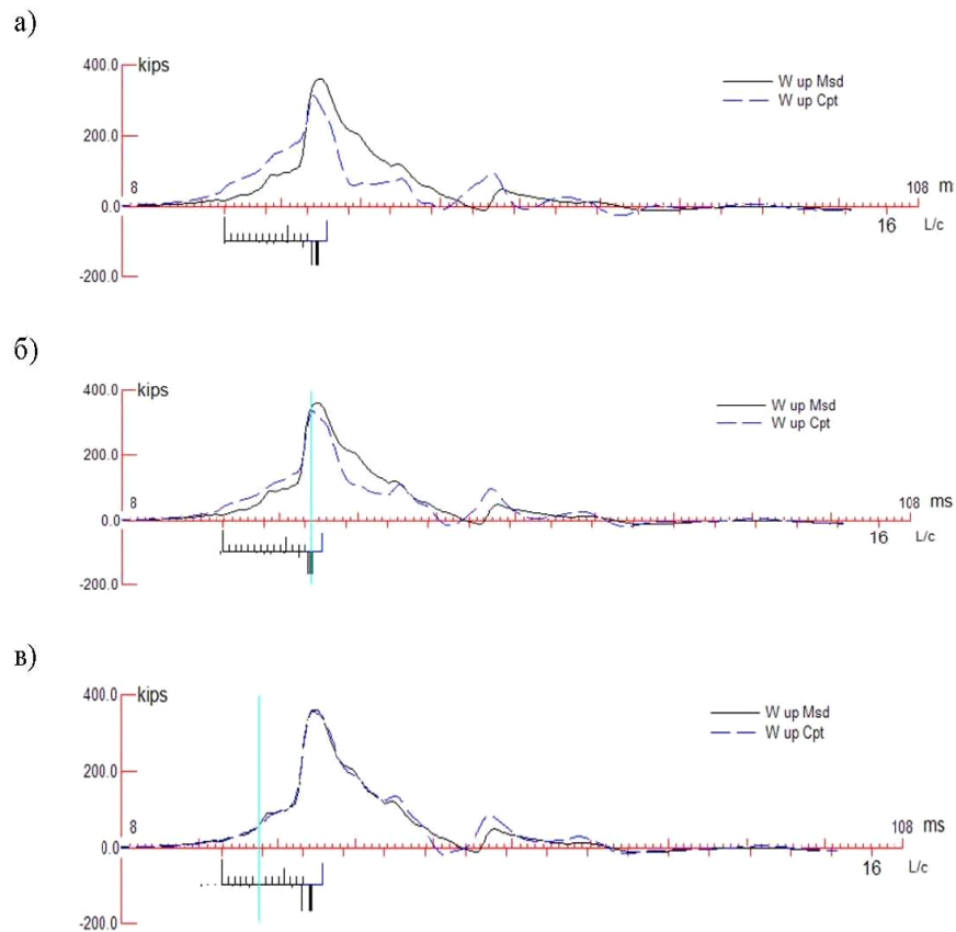
Д.13-сурет – «Салыстыру» есепті және өлшенген қисық CAPWAP
