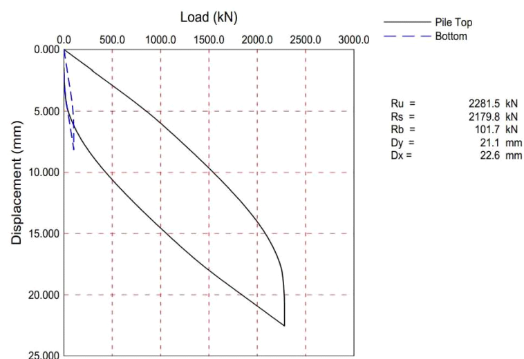
Д.14-сурет – PDA әдіс сынаулар нәтижелер бойынша «жүктеме-тұнбалық» кесте
